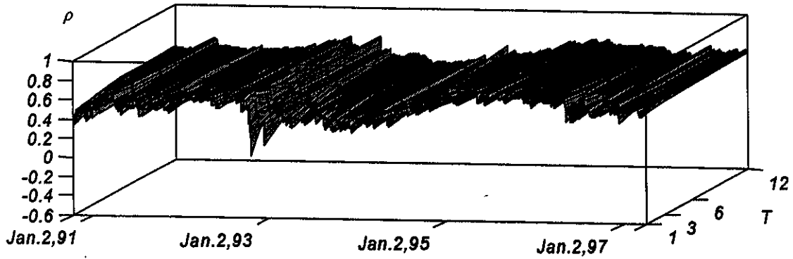
B. \rho(USD_{DEM}, JPY_{DEM})
